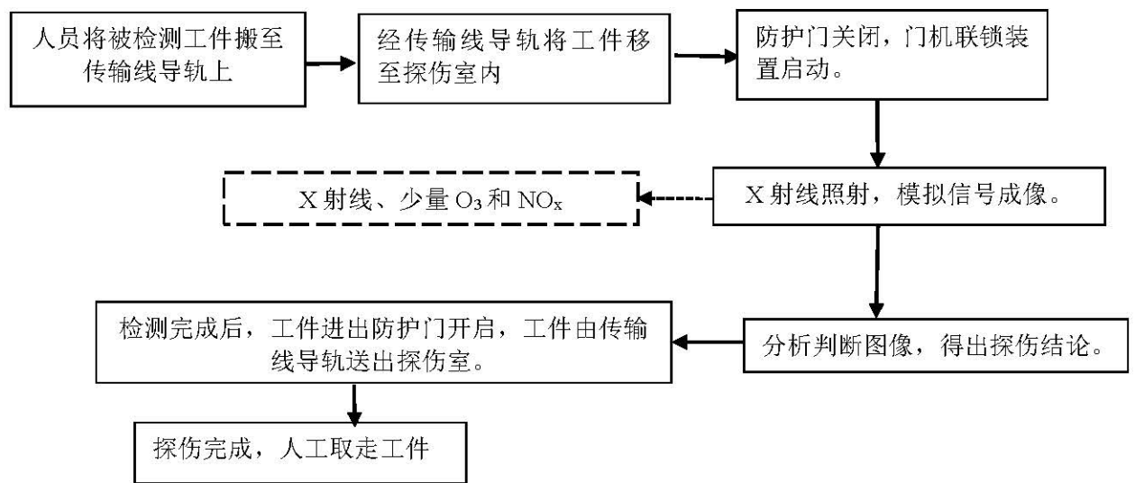
图 9-2 X 射线数字成像检测系统探伤工作流程及产污环节示意图
